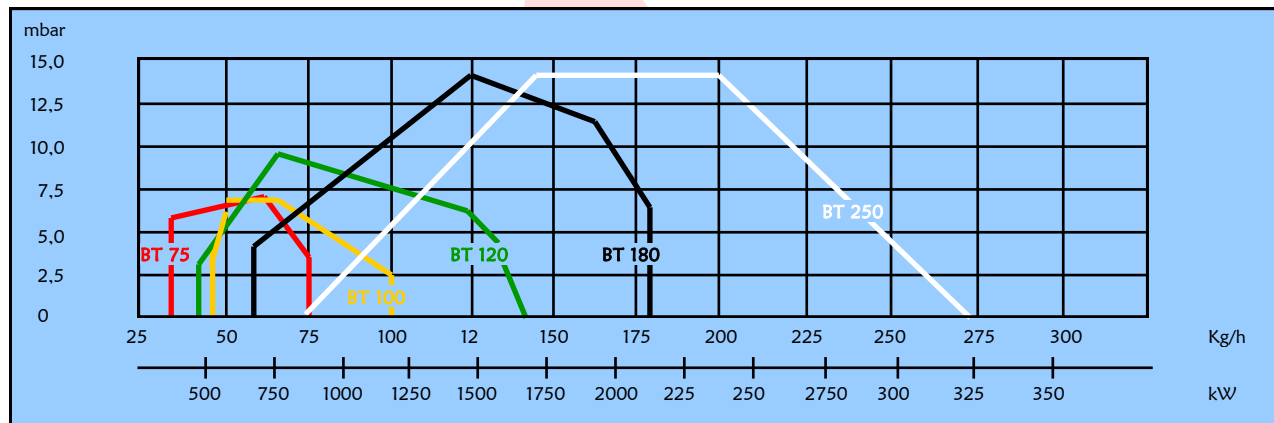
Kapacitetsdiagram
